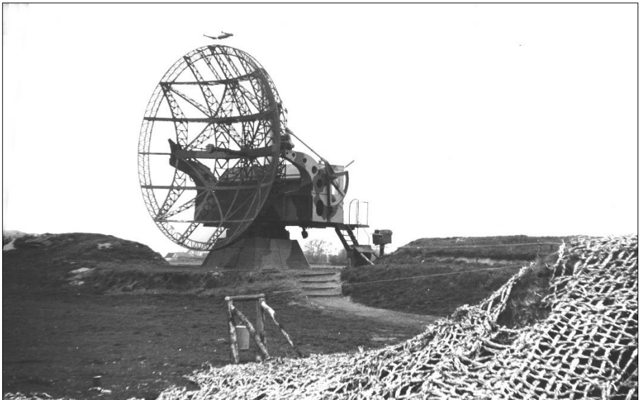
Tysk Luftwafferradar af typen Würzburg Riese opstillet 1942. Fotoudlån: Frihedsmuseet.
